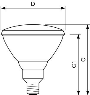
PAR38COL 80W E27 230V BL
